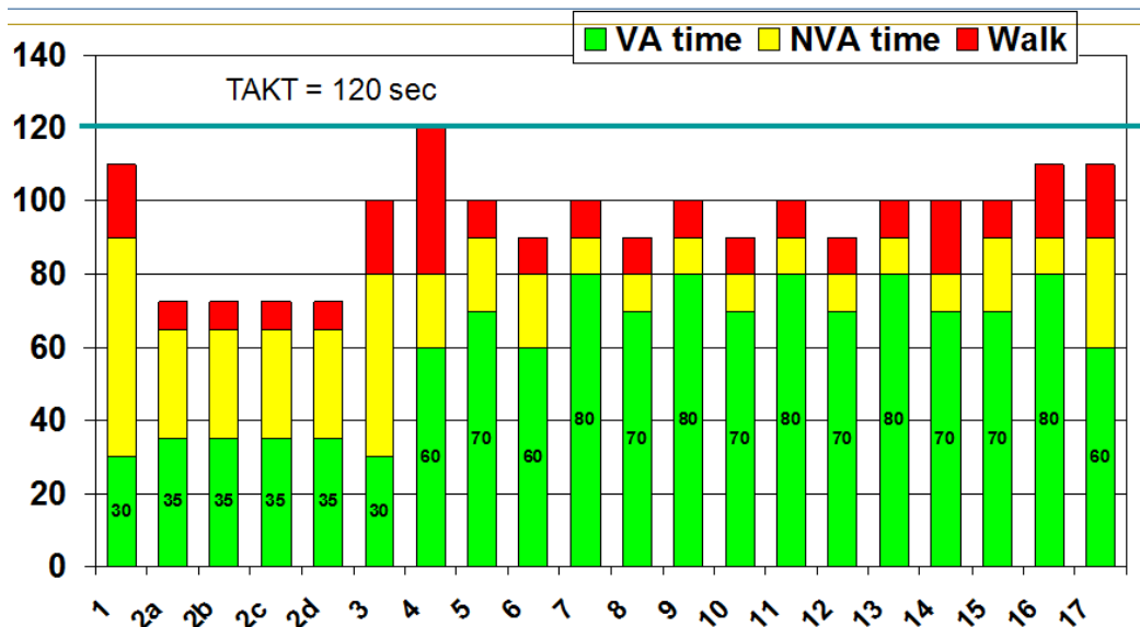
Figura 2.7 – Load chart que representa a cronoanálise das operações do processo.
