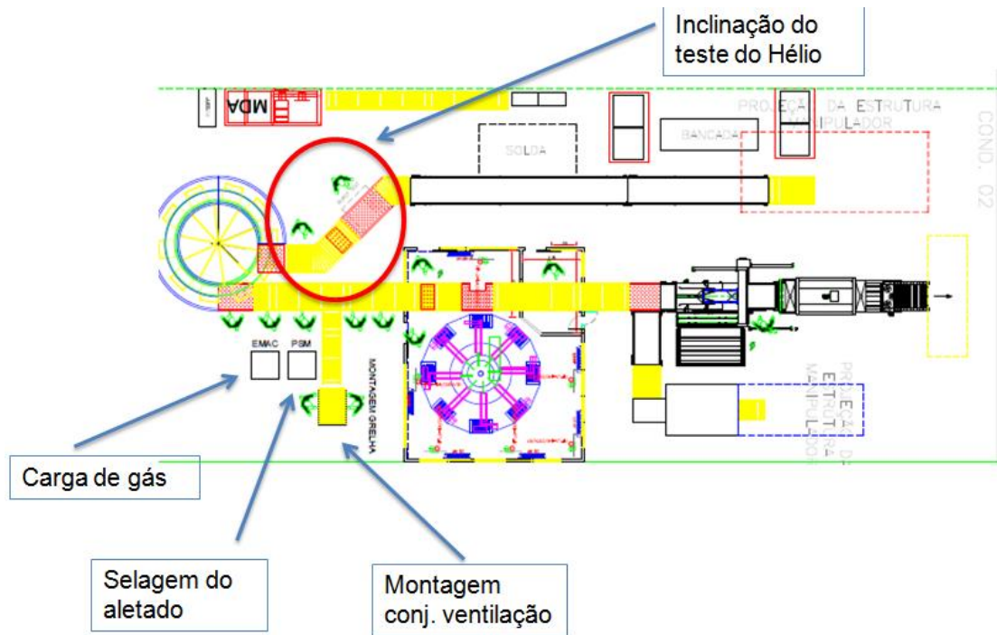
Figura 4.10 – Layout definido para suprir o aumento de capacidade da linha.
