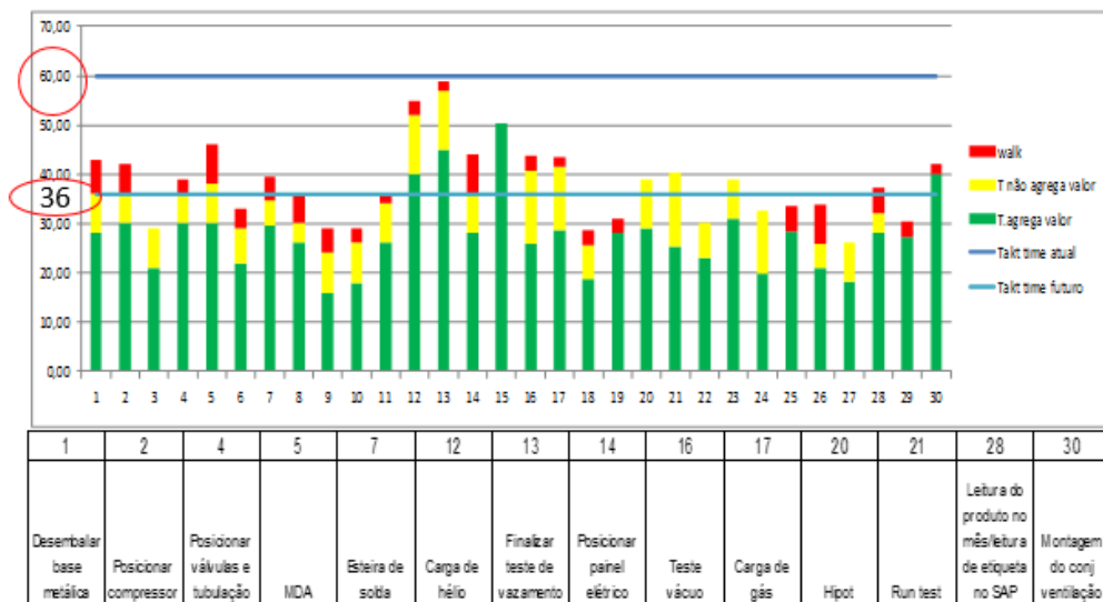
Figura 4.4 – Load Chart do processo.
