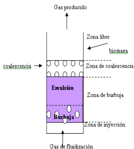
Figura.1. Zonas diferenciadas en el gasificador de LF.
