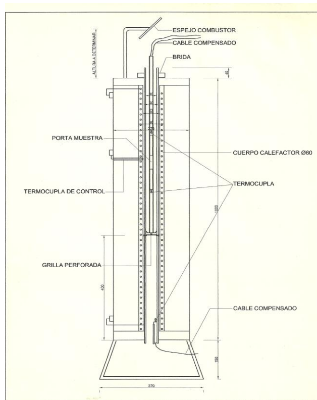
Figura 1. Diagrama del reactor tubular empleado en las experiencias
